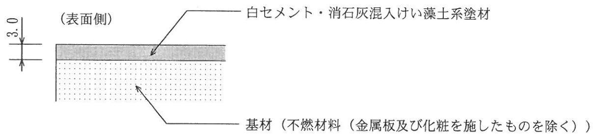
図1 断面図
