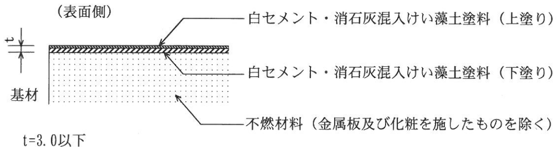
図1 断面図
